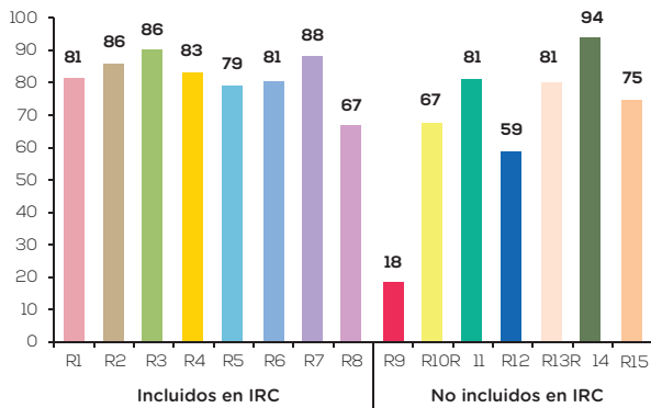
Valores IRC LED estándar (IRC 82)
